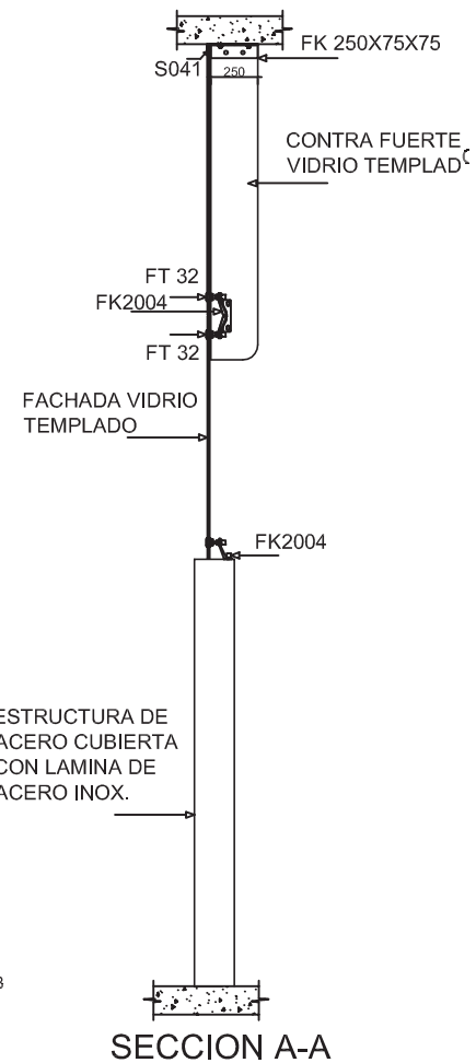
FACHADA VIDRIO TEMPLADO
