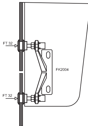
ELEVACION FRONTAL
