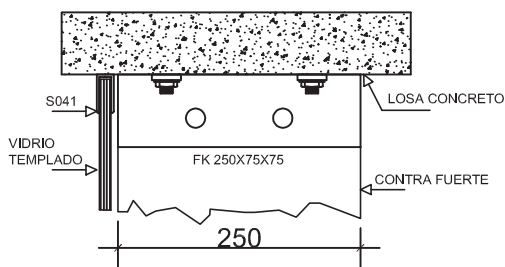
ELEVACION FRONTAL
