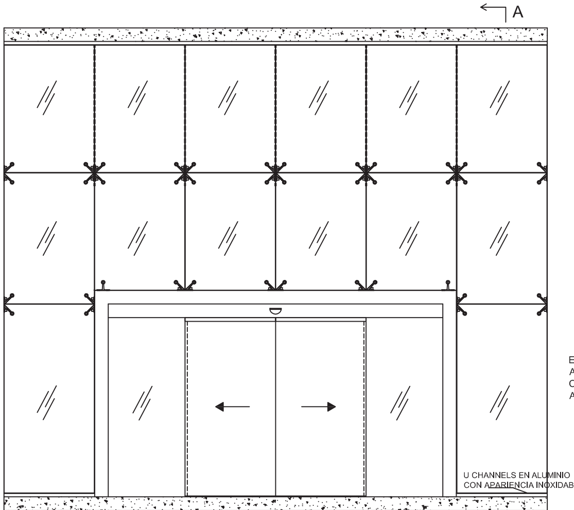
ELEVACION FRONTAL
