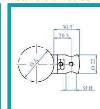
Detalle diametros
