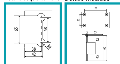
Detalle saque/barreno Detalle Medidas
