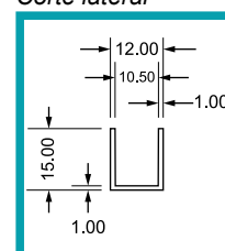
Corte lateral
