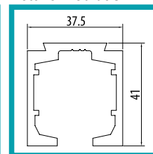
Detalle medidas
