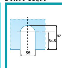
Detalle Saque
