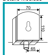
Detalle Medidas
