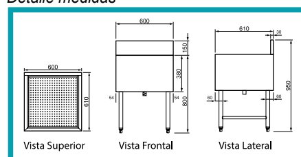
Detalle medidas
