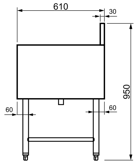
Vista Lateral
