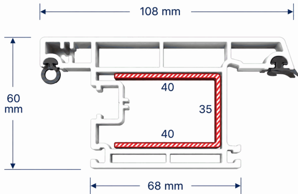
Sección - Perfil uPVC Hoja de Puerta Apertura Exterior - Serie 60 mm
