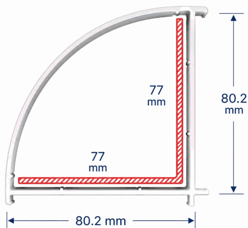
Sección – Perfil uPVC Adaptador Unión de Esquina de 80/80 mm
