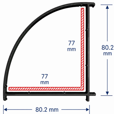
Sección – Perfil uPVC Adaptador Unión de Esquina de 80/80 mm
