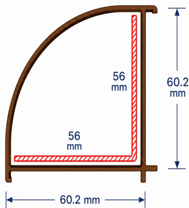
Sección - Perfil uPVC Adaptador Unión de Esquina de 60/60 mm
