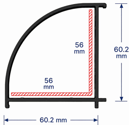
Sección - Perfil uPVC Adaptador Unión de Esquina de 60/60 mm
