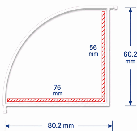
Sección – Perfil uPVC Adaptador Unión de Esquina de 80/60 mm
