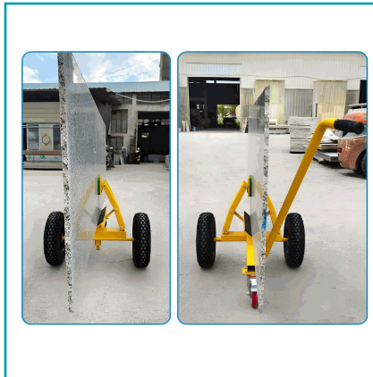
Bocanilla de inflado de neumáticos. Rueda de goma elástica / Inflado fácil y sin esfuerzo.
