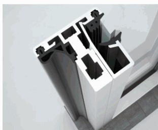
Conexión Paño Fijo/ Recibidor Puerta
