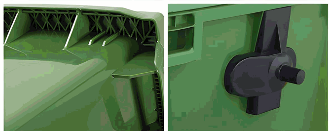
REFUERZO EN EL BORDE DEL BARRIL
